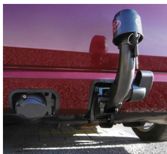
Фаркоп з'ємний
